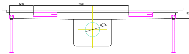
Front aanzicht
